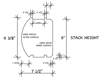
8x10 JUMBO D LOG
