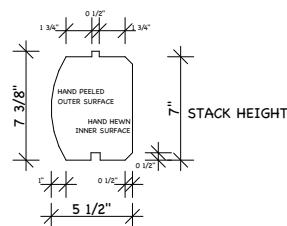
6x8 D LOG
